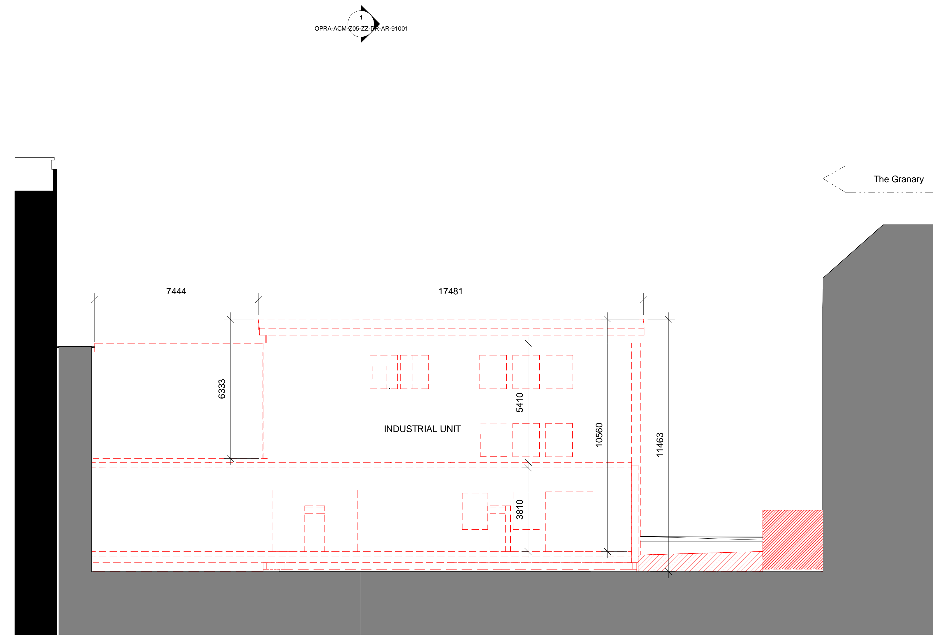
3 Section C-C Existing SCALE: 1 : 100
