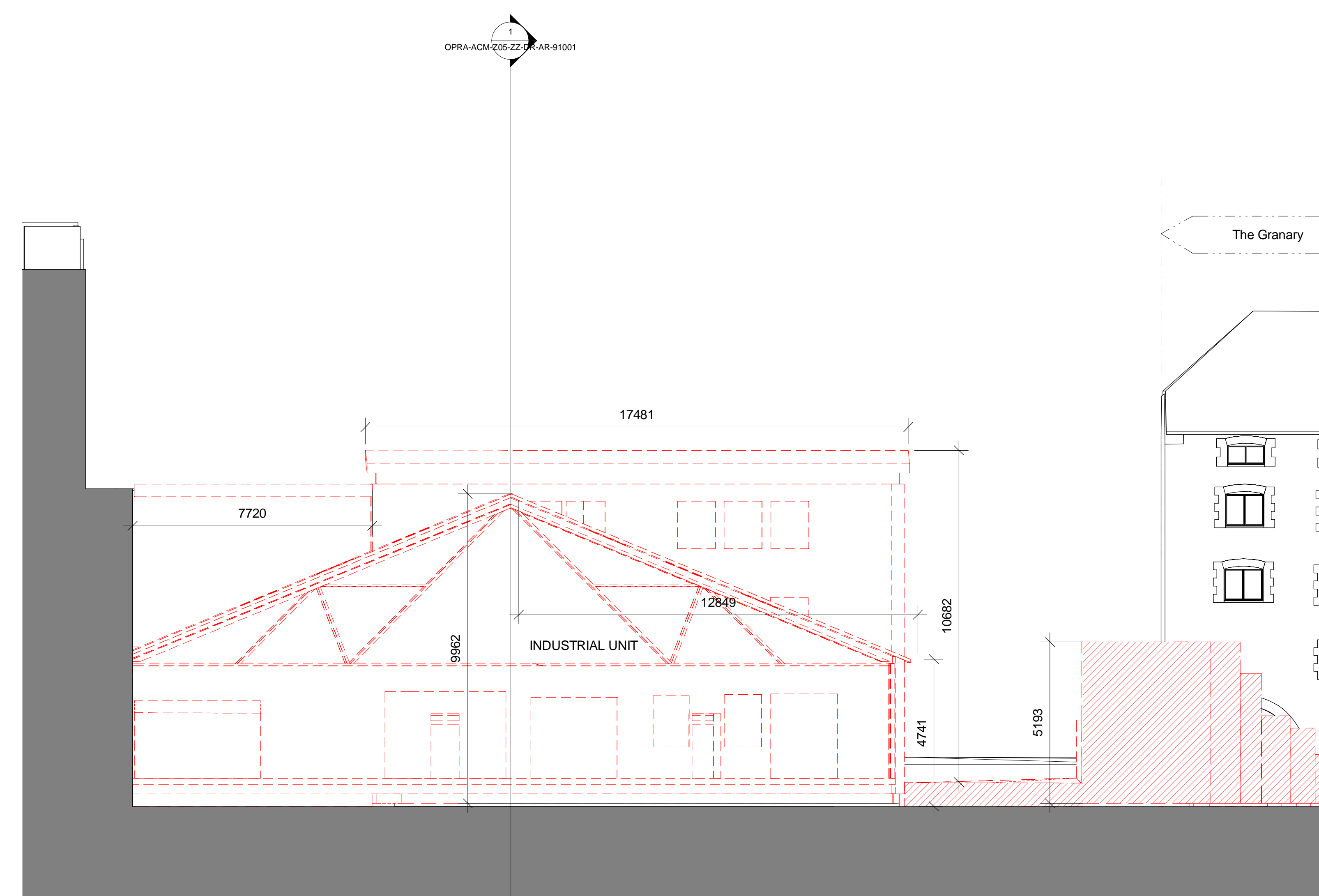
2 Section B-B Existing SCALE: 1 : 100
